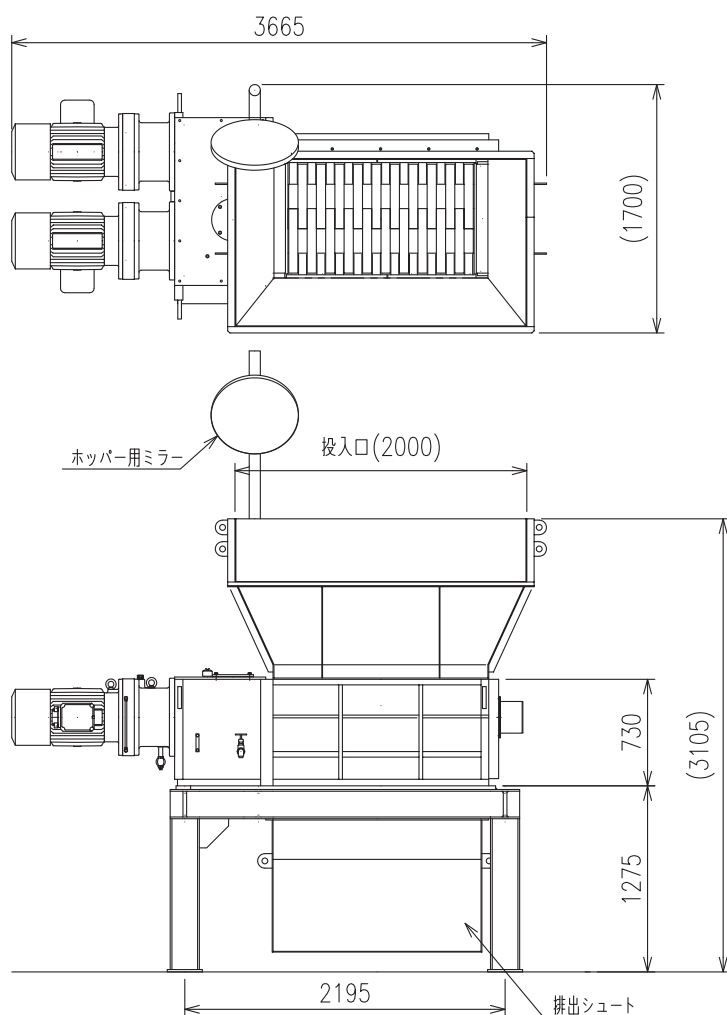
装置仕様
